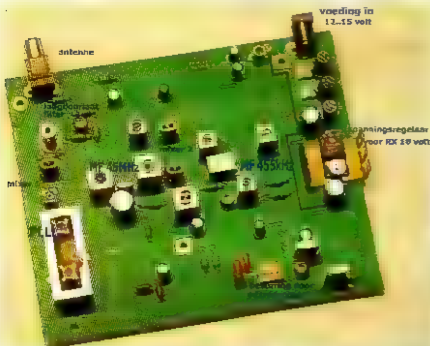
Ingangsgedeelte en middenfrequent van de RX-320.
